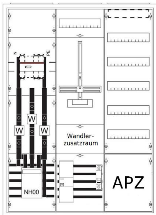
Abbildung 3: Beispielhafter Aufbau einer halbindirekten Messung bis 100 A Betriebsstrom (Höhe min. 1050 mm)
