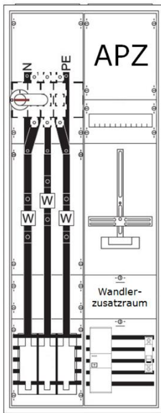
Abbildung 4: Beispielhafter Aufbau einer halbindirekten Messung bis 250 A Betriebsstrom (Höhe min. 1350 mm)
