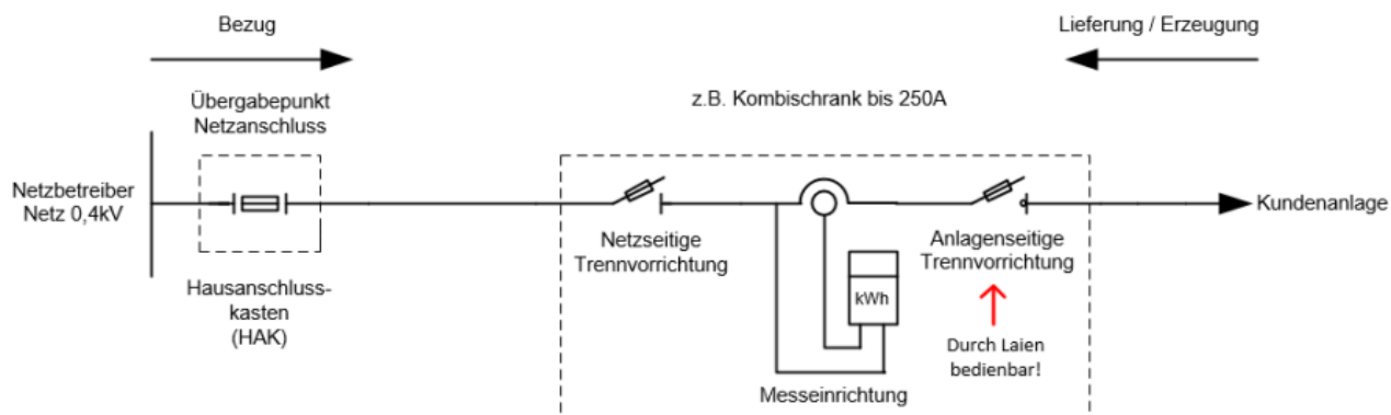
Abbildung 2: Prinzipielle Darstellung der netzseitigen- und anlagenseitigen Trennvorrichtung
