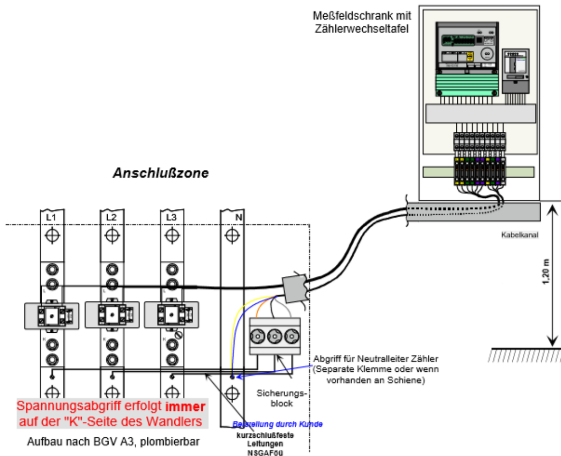
Abbildung 8: Schema möglicher Anschluss mit Zähler, Niederspannung
