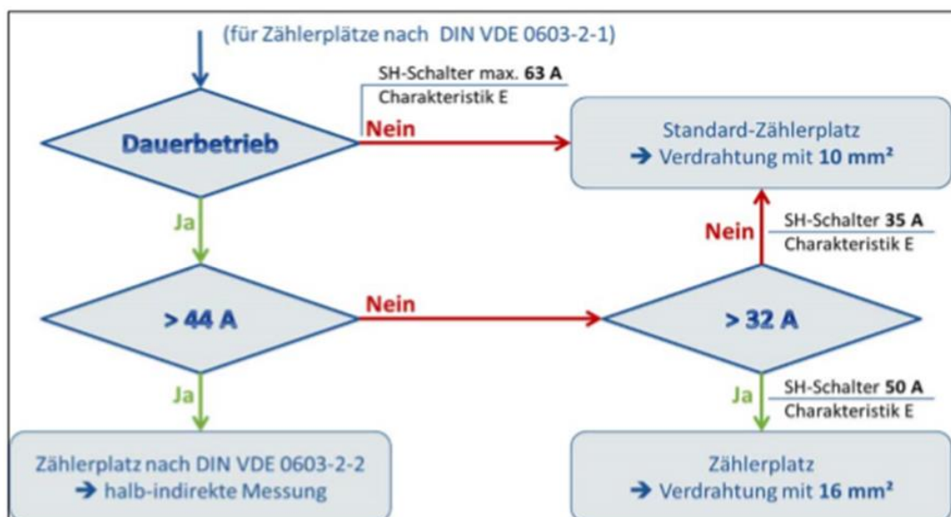
Abbildung 1: Vereinfachte Darstellung der Belastungs- und Bestückungsvarianten von Zählerplätzen
