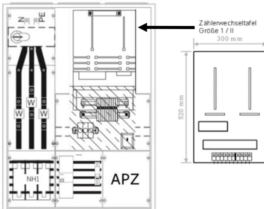
Abbildung 5: Beispielhafter Aufbau einer halbindirekten Messung (Wandlermessung) ab 250 A Betriebsstrom
