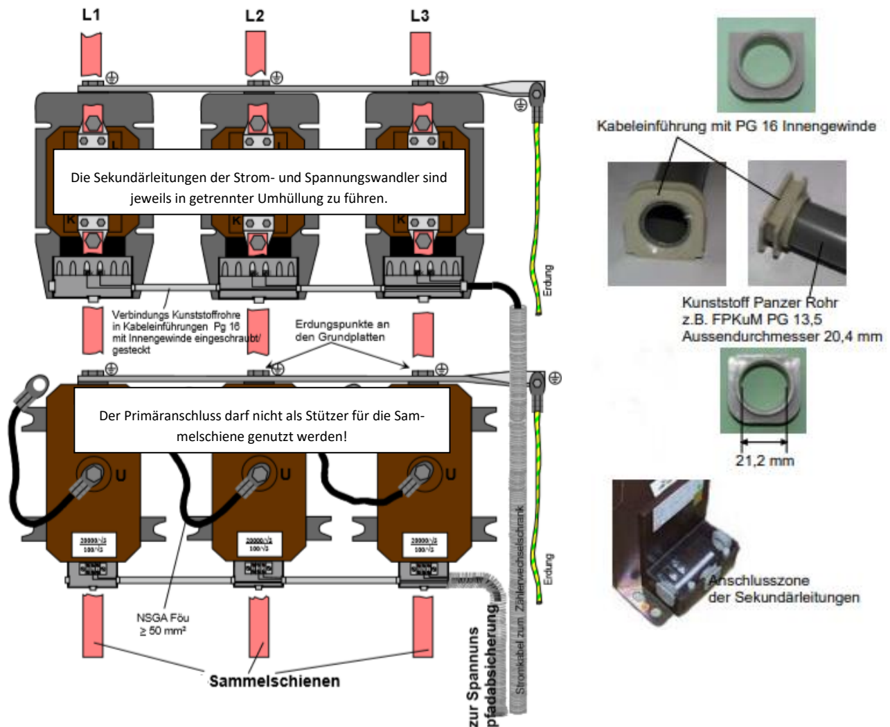
Abbildung 10: Schema mögliche Anordnung Strom- und Spannungswandler, Mittelspannung
